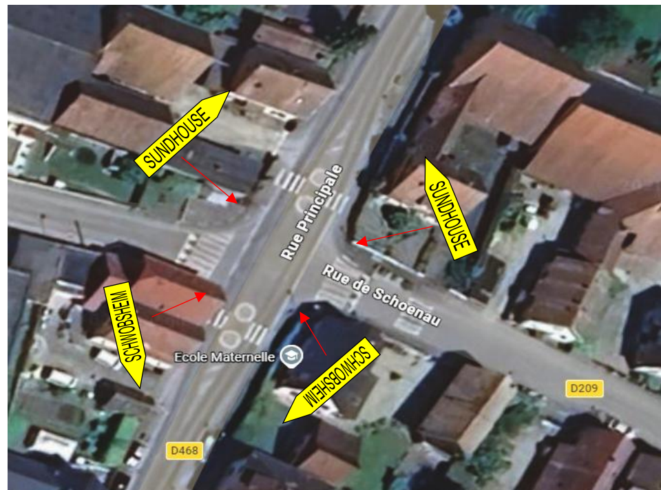
détail 4: Richtolsheim; intersection D468 / D209
